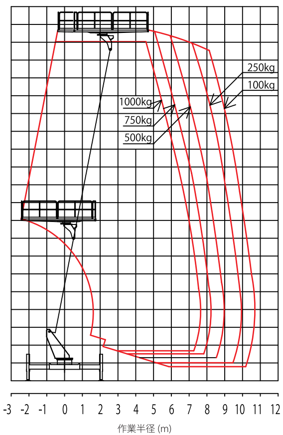
アウトリガ中間 2 張出
