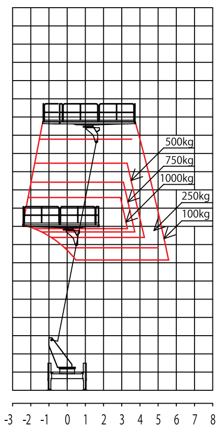
アウトリガ最小張出
