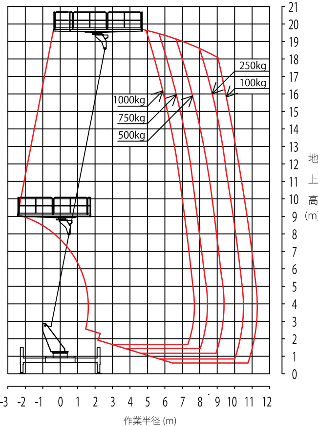
アウトリガ最大張出
